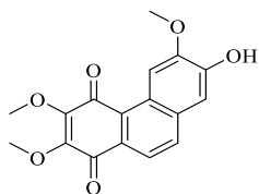
Combretastatin C-1
