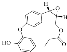
Combretastatin D-1
