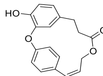
Combretastatin D-2
