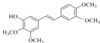
Combretastatin A-6
